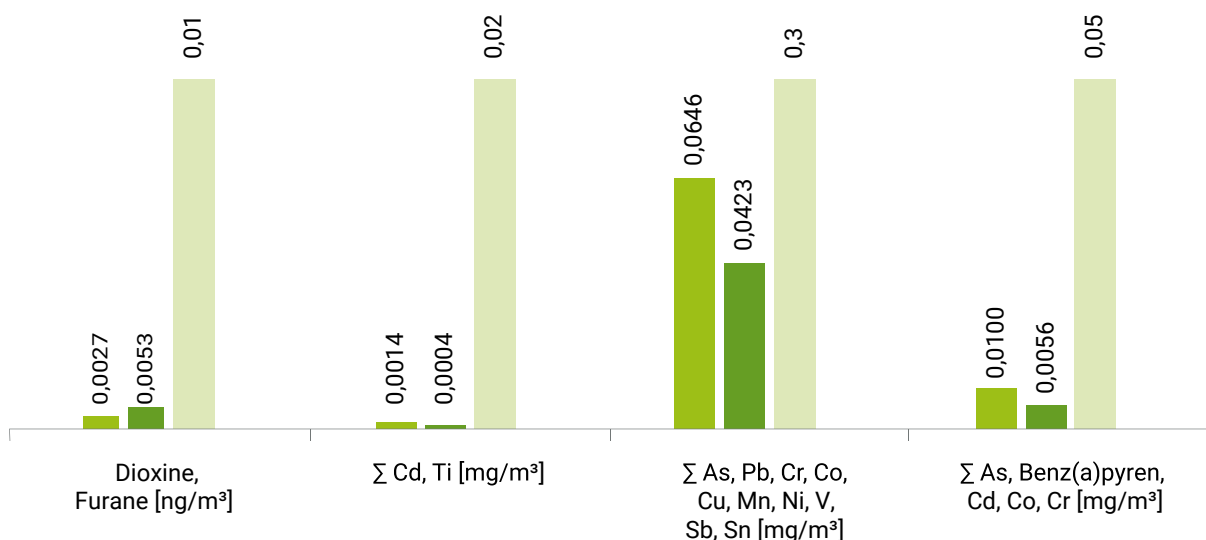
Mittelwerte der Einzelmessungen vom DHE im Jahr 2025: Linie 1 | Linie 2 | Grenzwerte
