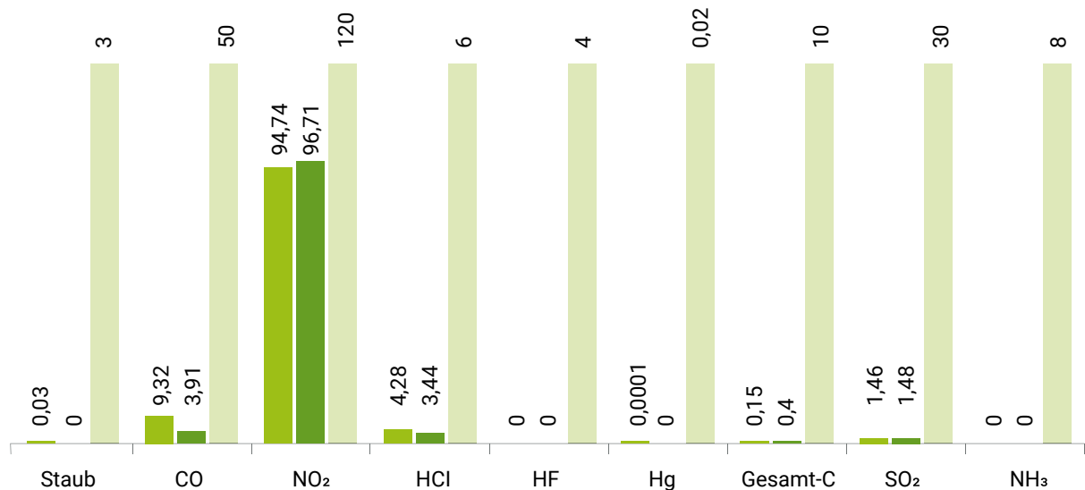
Durchschnitt aller Tagesmittelwerte der DHE-Anlage in 2025 [mg/m³]: ■ Linie 1 ■ Linie 2 ■ Grenzwert als Tagesmittelwert [mg/m³]
